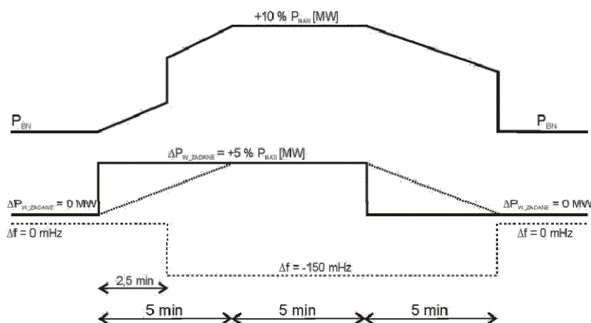
Rys. 8 Sprawdzenie współdziałania regulacji odbudowy częstotliwości oraz regulacji FSM
