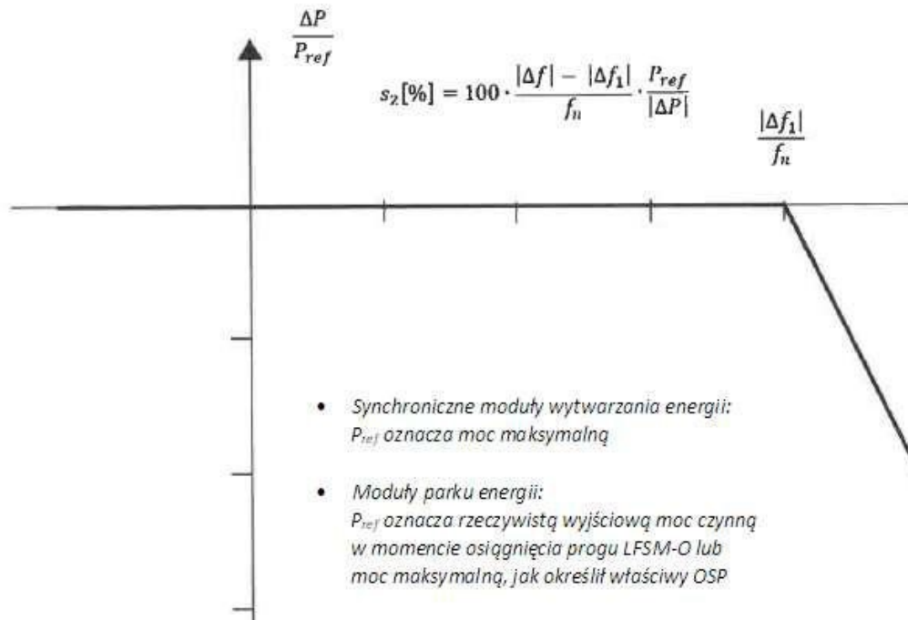
Rys. 1. Zdolność modułów wytwarzania energii do odpowiedzi częstotliwościowej mocy czynnej w trybie LFSM-O
